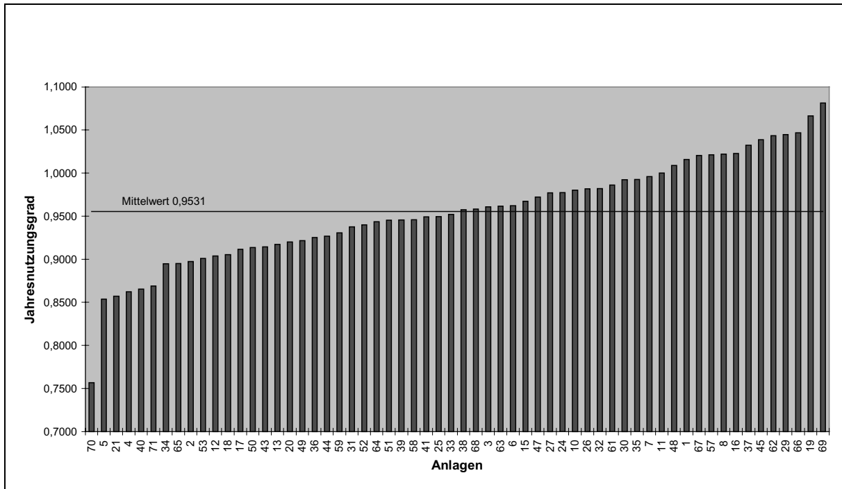
Bild 5 Messwerte für Nutzungsgrad von Brennwertkesseln
