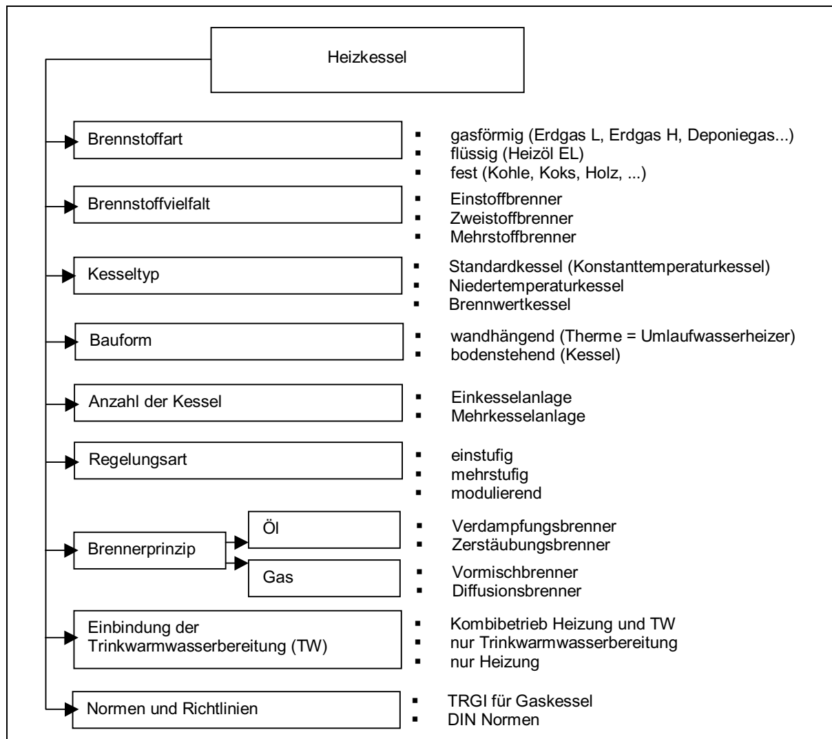
Bild 1 Einteilung der Heizkessel
