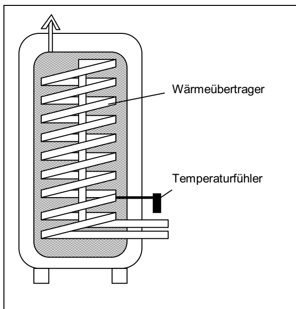
Bild 7 Indirekt beheizter Trinkwarmwasserbereiter
