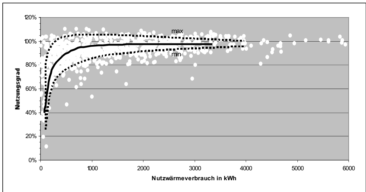
Bild 6 Messwerte für Nutzungsgrad je nach Kesselauslastung
