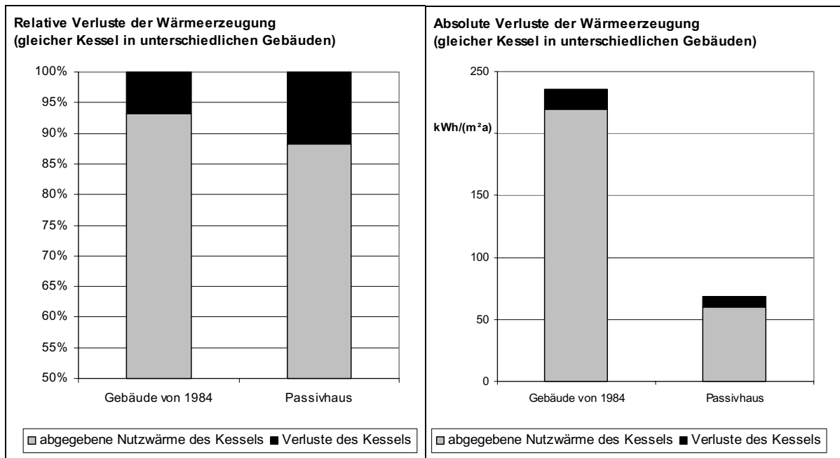
Bild 4 Nutzungsgrad und Erzeugerverluste für unterschiedliche Gebäude
