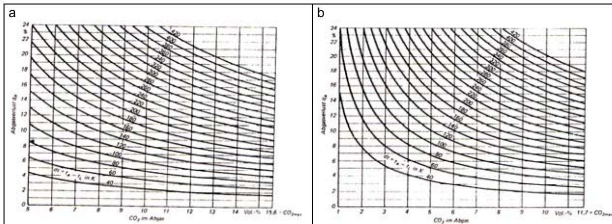
Bild 2 Abgasverluste für die Verbrennung von Erdgas (a) und Heizöl EL (b)
