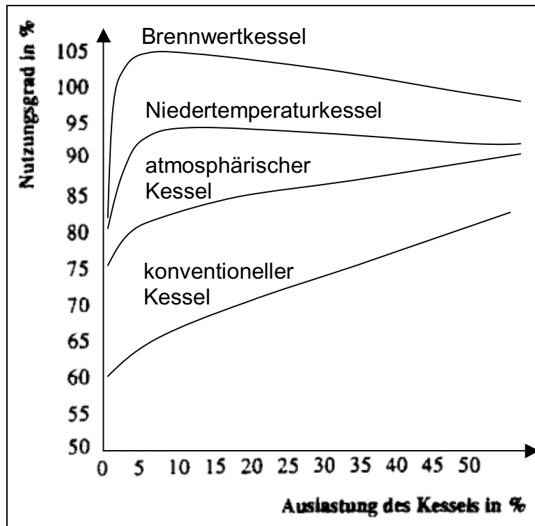
Bild 3 Nutzungsgrad nach Kesselprinzip (schematisch)
